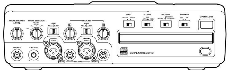
Frente. Grabador de CD-R/CD/RW, Entrada de micrófono y línea (XLR y 1/4"), Salida de auriculares (1/4") [Headphone OUT].
