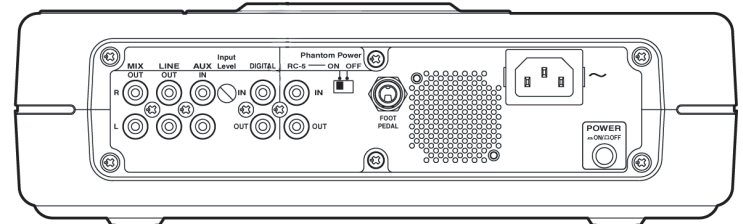
Atrás. Entrada Digital RCA [IN/OUT] (S/PDIF), entrada de pedal (1/4") [Foot Pedal IN], entrada auxiliary [AUX IN].
